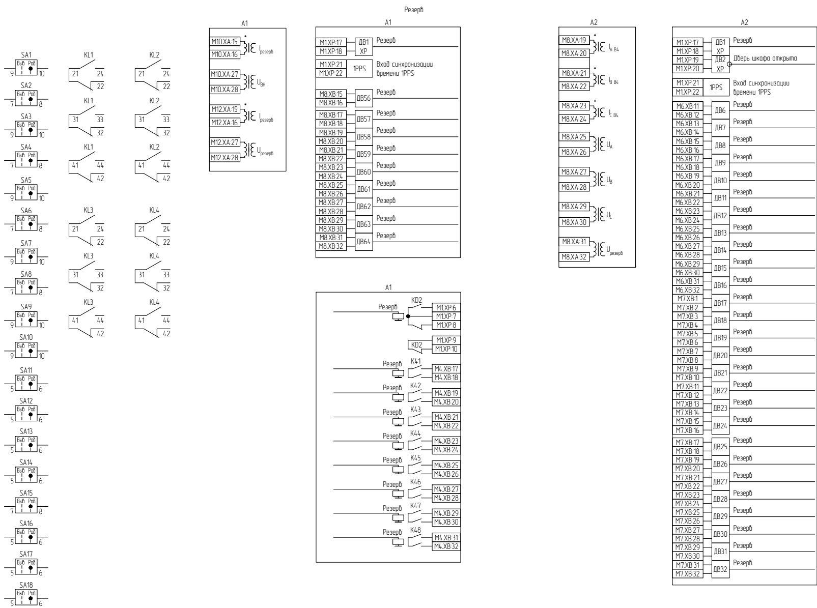
Рисунок В.10 – Схема электрическая принципиальная (часть 10)
