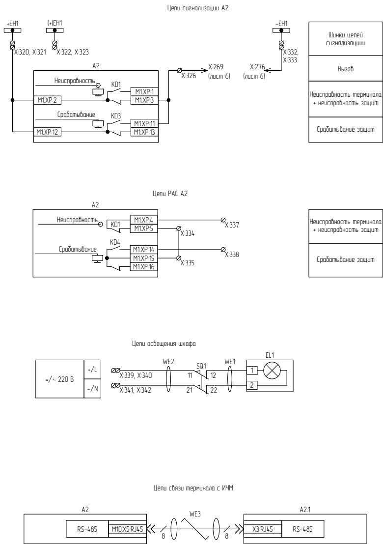
Рисунок В.9 – Схема электрическая принципиальная (часть 9)
